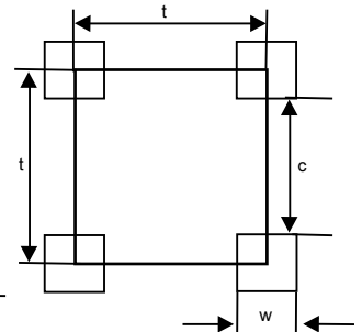
QG Quadratlochung in geraden Reihen
